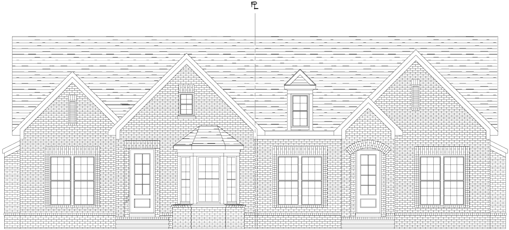
Elevation A*
