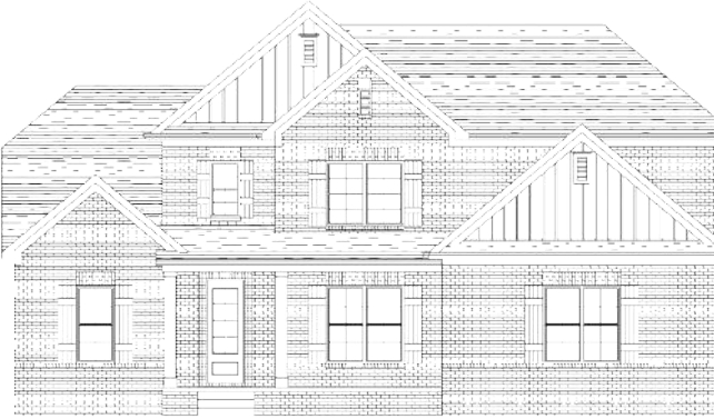
Elevation B
